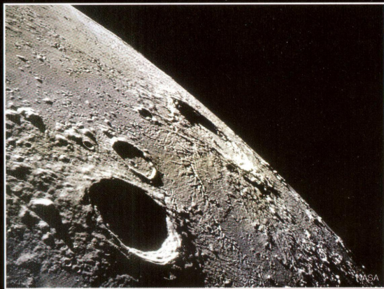
月面には無数のクレーターがあります。 その中で、コペルニクスというクレーターは新しいものです。
