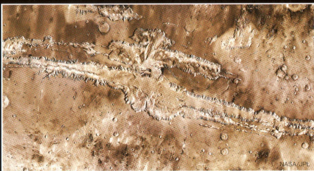
火星大地の裂け目、マリネリス峡谷(長さ4000km)です。 極地方では、水(氷)も見つかっています。
